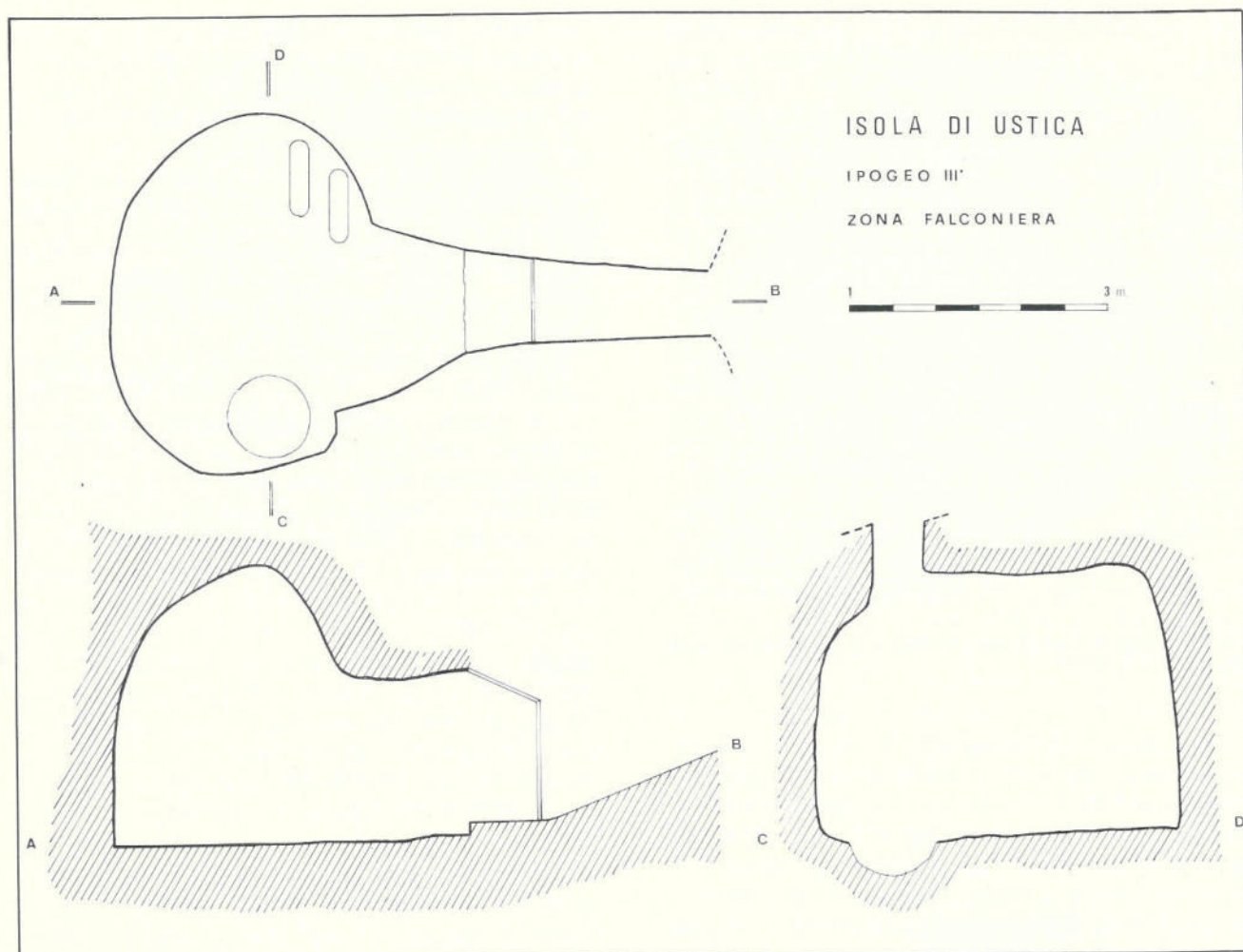
FIG. 25 - Ustica. Falconiera, Tomba ipogeica IV: pianta e sezioni (G. Vella).
